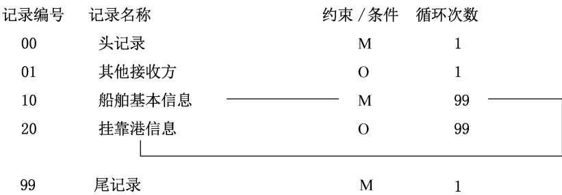
图 5 文件结构
